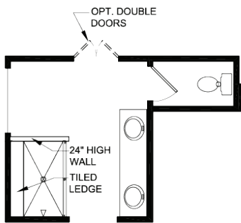
OPTIONAL DELUXE SHOWER
